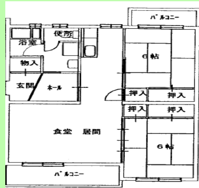
間取り図(一部)
